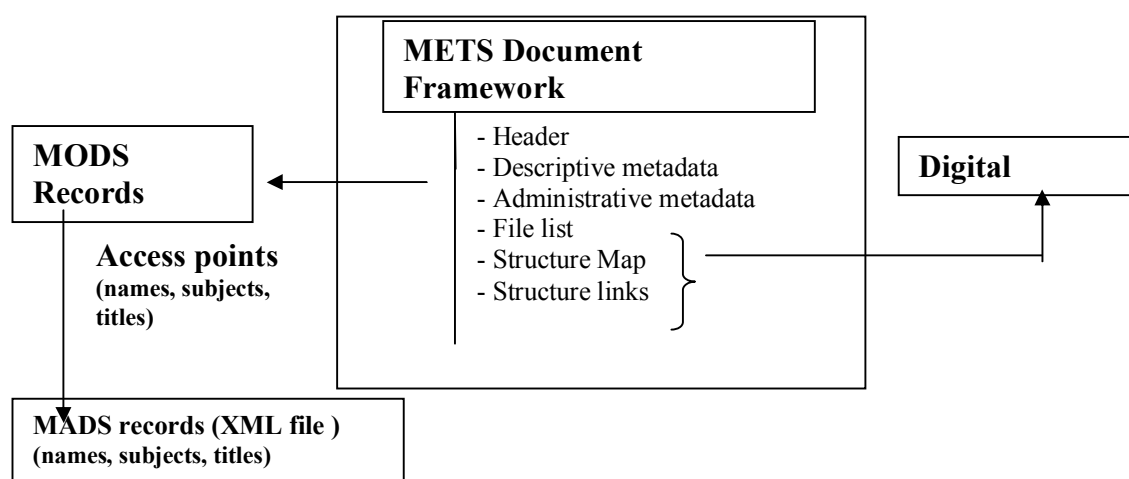
แผนภาพที่ 3 ความสัมพันธ์ของ MODS record, METS Document Framework, และ MADS record บนโปรแกรม Greenstone Digital Library Software
